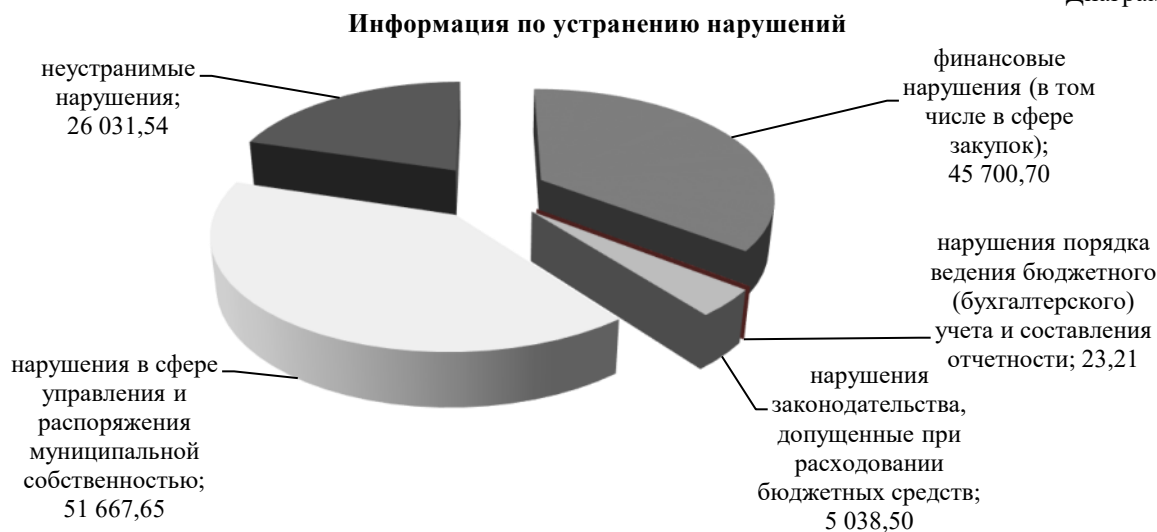
Диаграмма №3
