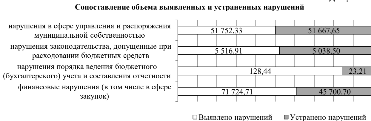
Диаграмма №4
